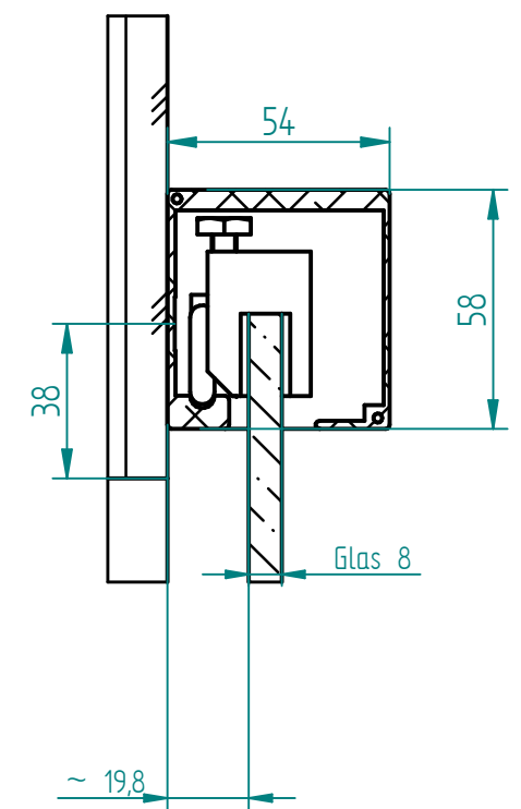
EINZELHEIT B
